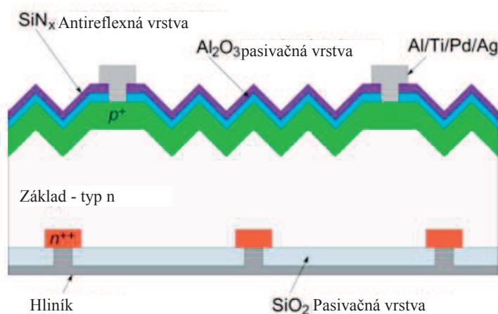
Obrázok 2 Štruktúra bunky s borovým rozptýleným čelným emitorom [11]
